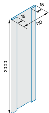
Plochý podkladový profil tloušťka: 0,65 mm - délka: 2 m
