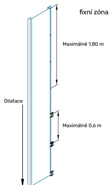
Standardní pokládka vertikální
