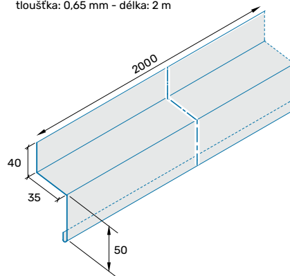
Lemovací profil tloušťka: 0,65 mm - délka: 2 m
