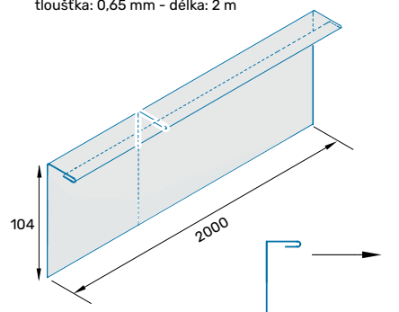
Ukončovací profil tloušťka: 0,65 mm - délka: 2 m
