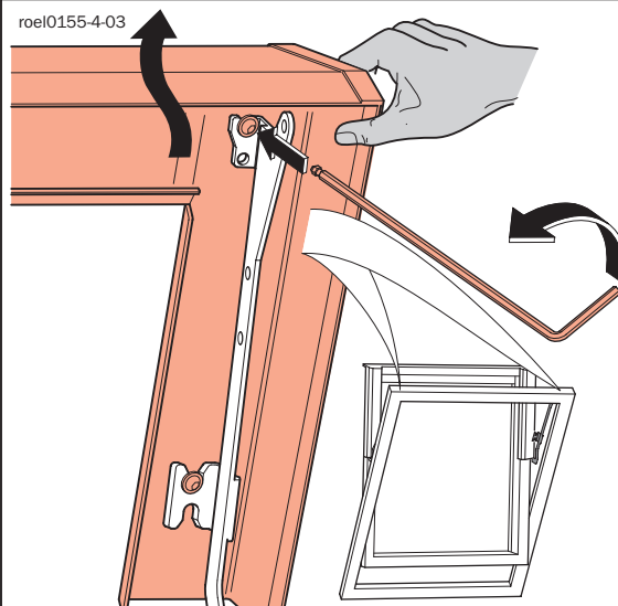
Flügelblech demontieren
