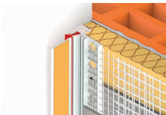
Lišta s tkaninou 9 mm 3D PRO s těsnícím jazýčkem
