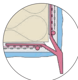
Zakončovací profil s přiznanou okapnicí
