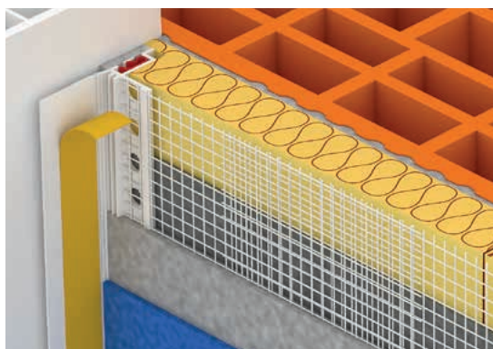
Lišta s tkaninou FAP Compact 3D PRO
