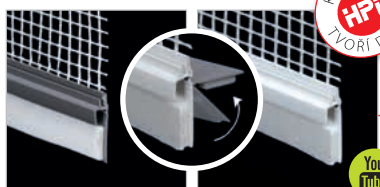
Detail aplikace připojovacího profilu parapetního
