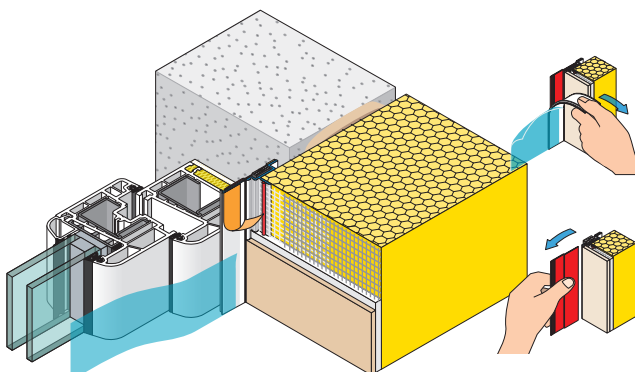
Lišta s tkaninou PUR-FIX-pro
