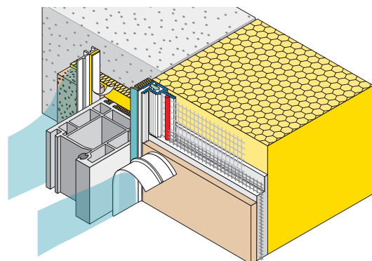
Lišta s tkaninou teleskopická s jazýčkem
