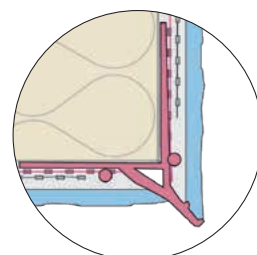
Zakončovací profil s okapnicí pod omítku
