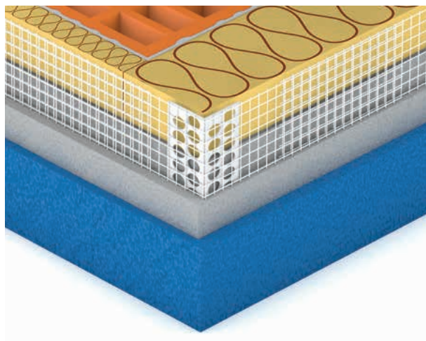
Applikace kombi lišty s tkaninou
