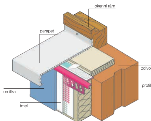
Detail aplikace připojovacího profilu parapetního
