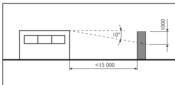
Výška komína u nástavby na ploché střeše
