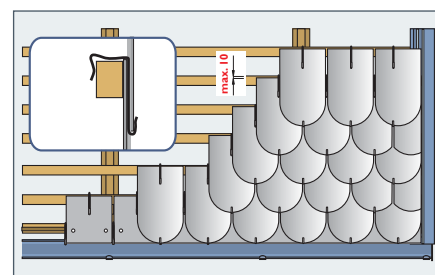
Montáž bobrovky - dvojité krytí
