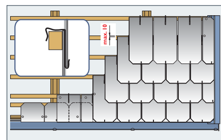
Montáž obdélníku - dvojité krytí
