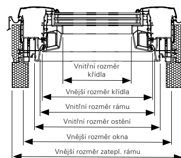
řez B-B
