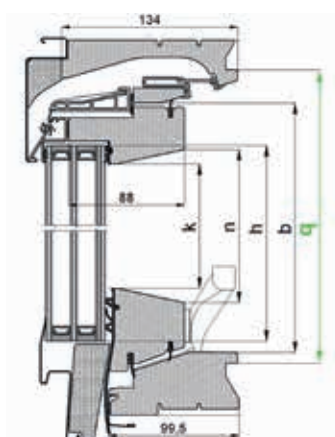
Délka SDK drážky v mm (q)
