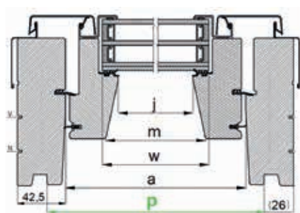
Šířka SDK drážky v mm (p)
